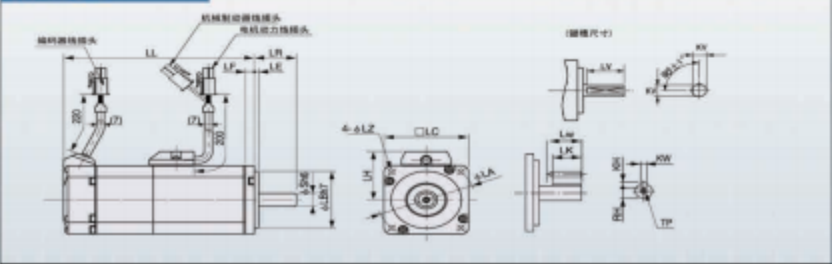
外形尺寸图
